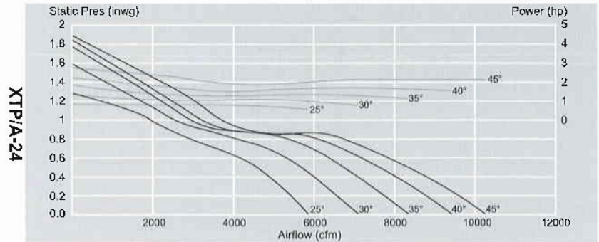
CURVAS DE OPERACIÓN (PERFORMANCE CURVES)
