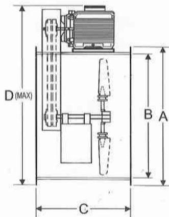
DIMENSIONES GENERALES (DIMENSIONS)
