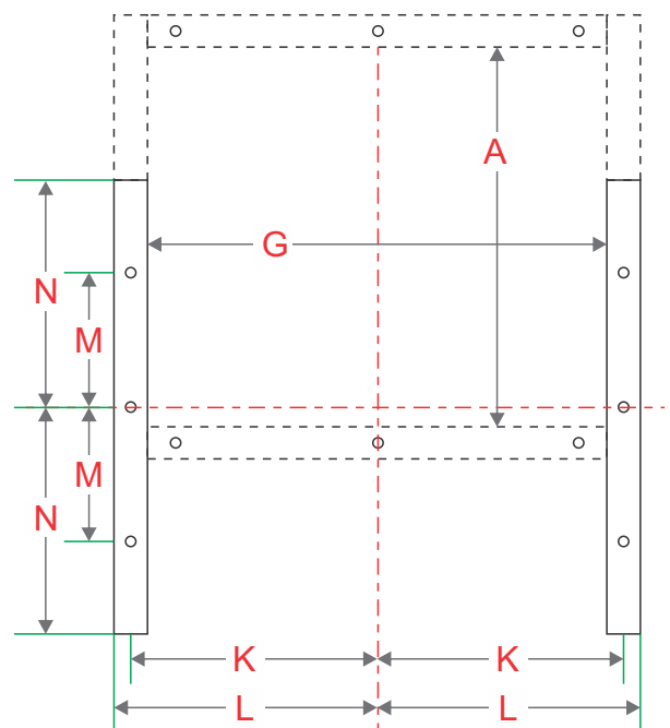
Vista planta para barrenos Foundation plan
